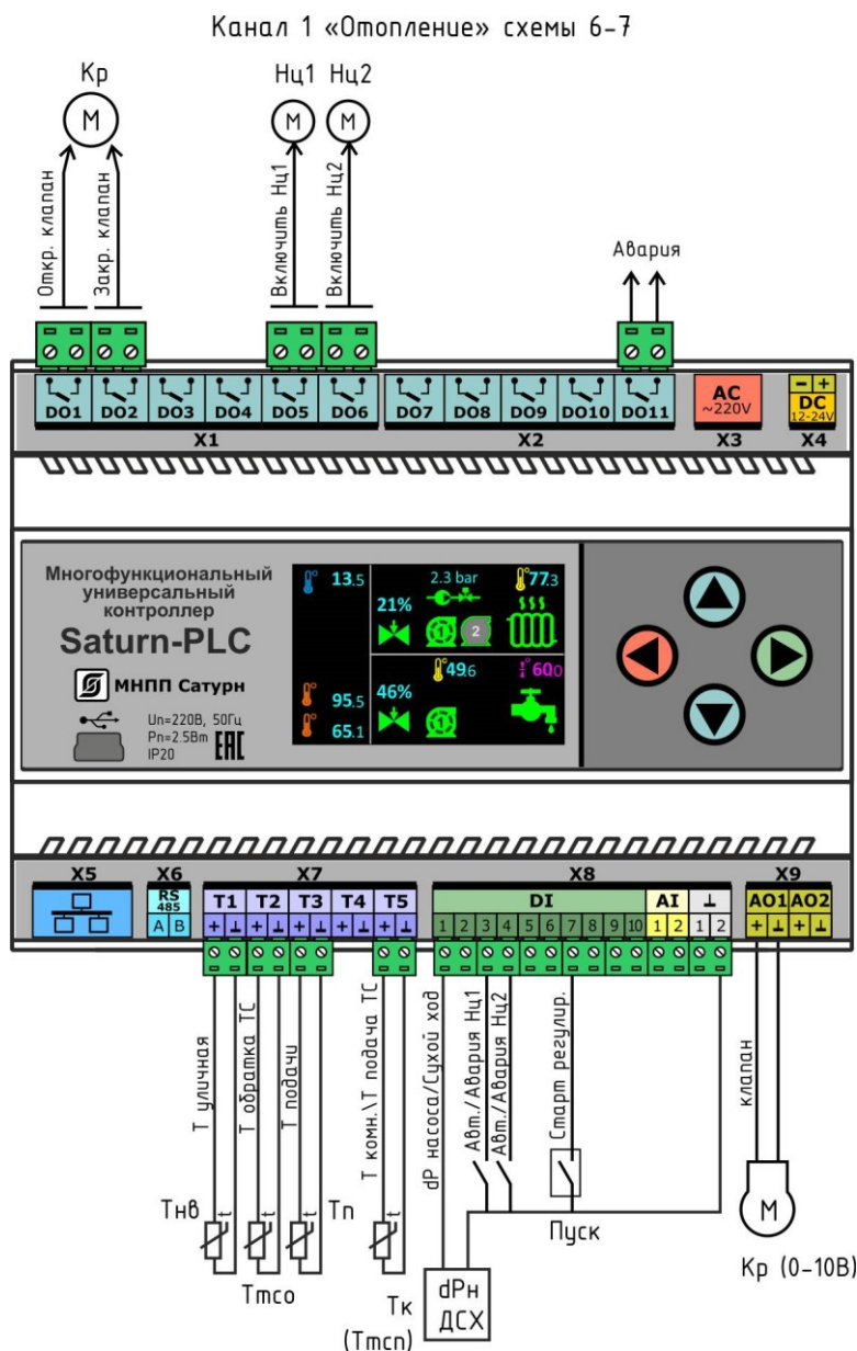
Рисунок 13 - Функциональная схема контроллера в режиме «Зависимое отопление», канал регулирования №1
