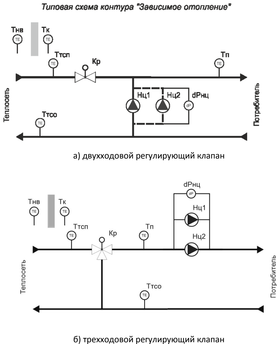
Рисунок 12 - Функциональные схемы контура отопления для зависимых схем
