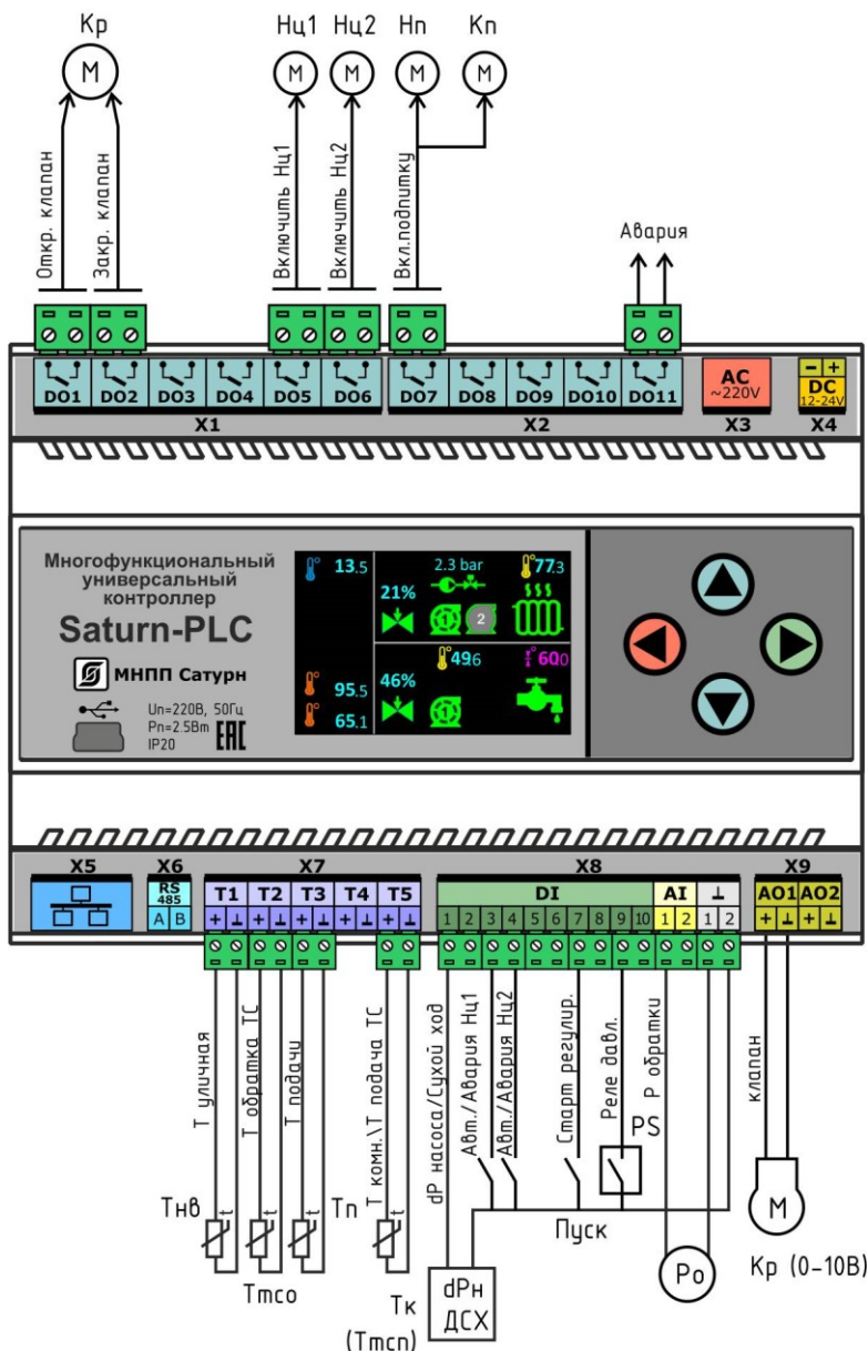
Рисунок 8 - Схема подключения датчиков и исполнительных механизмов в режиме «Отопление» (схемы 1-4) для канала регулирования №1
